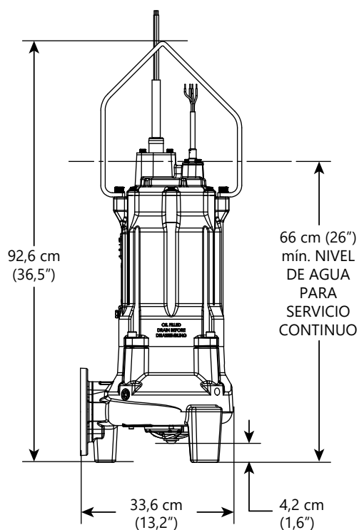
ANSI 150# de 2", 2,5" y 3" (DIN 50-PN10, DIN 65-PN10 y DIN 80-PN6) CON NPT DE 2"
