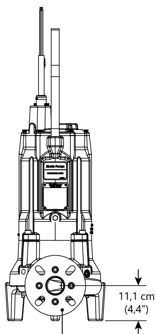
ANSI 150# de 2", 2,5" y 3" (DIN 50-PN10, DIN 65-PN10 y DIN 80-PN6) CON NPT DE 2"
