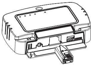
Figura 2. 9 V instalación de batería con bandeja
