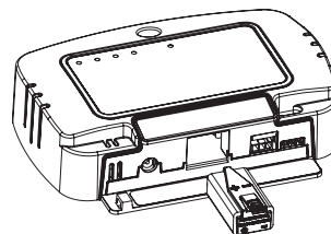
Figure 2. Installation de la pile 9 V avec plateau
